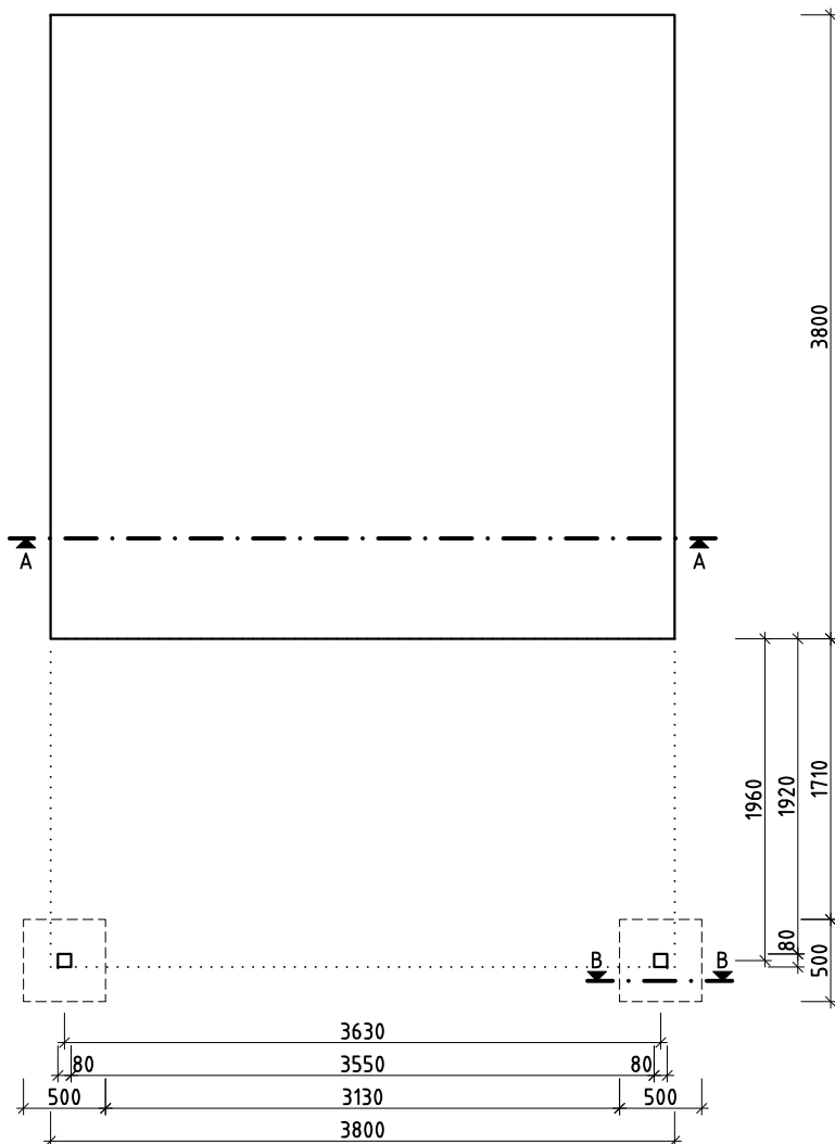
Fundament M 1:50
