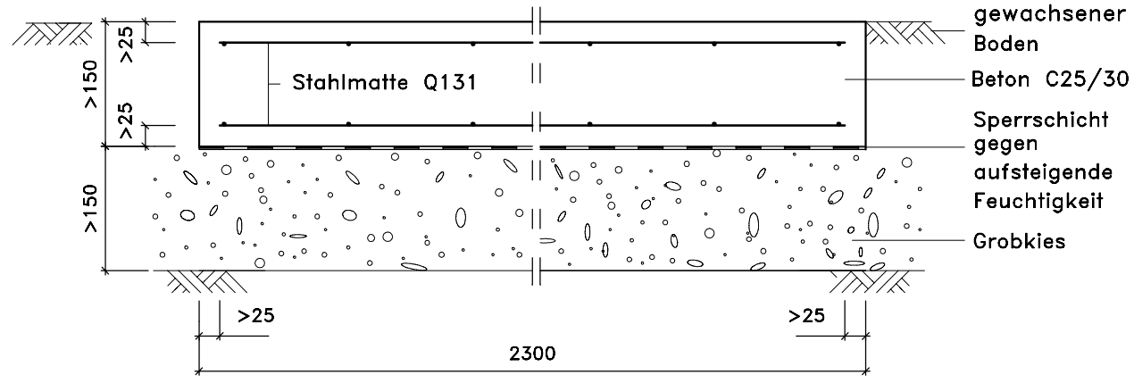
Schnitt A-A
