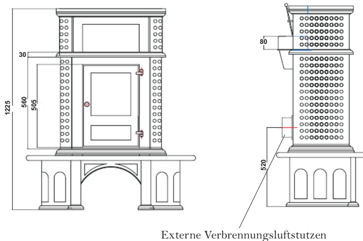
Externe Verbrennungsluftstutzen
